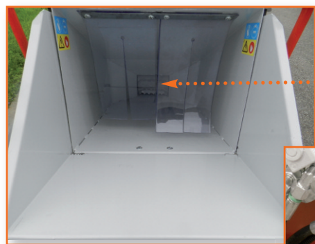
Montage avec 6 outils coupants fixes
